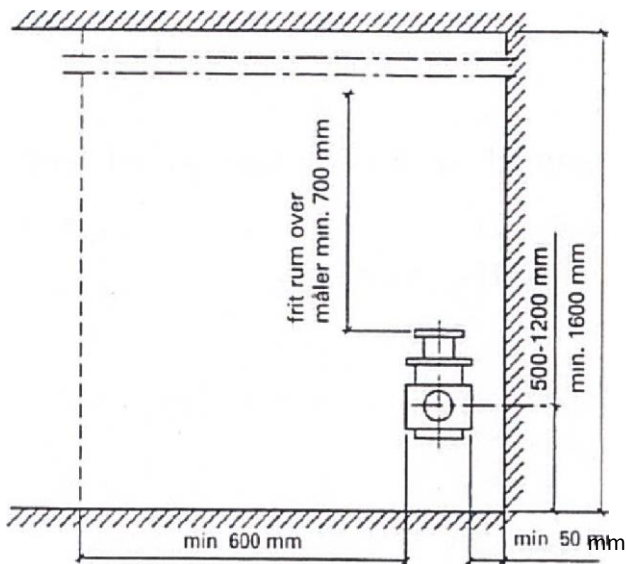
Figur 1 – Målerplacering jf. DS 439:2009, 3.5.2 i bygning med de frie afstande, der er nødvendige for aflæsning og udskiftning af måler.
